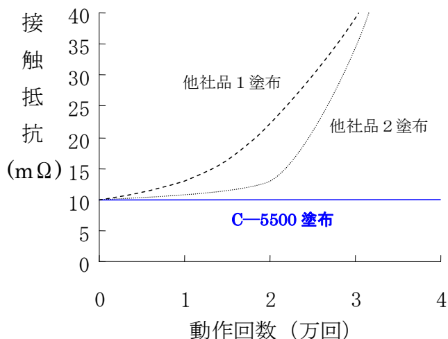
負荷寿命試験
