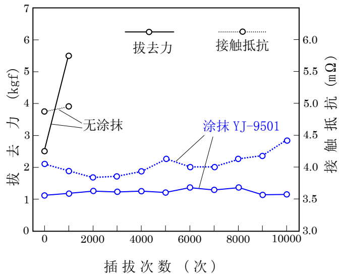
镀金接插件的插拔耐久试验
